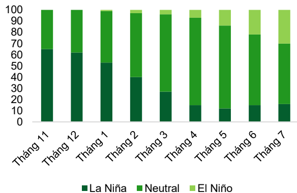
Xác suất xảy ra La Nina, El Nino, Trung lập từ T11/2025 -T7/2026
